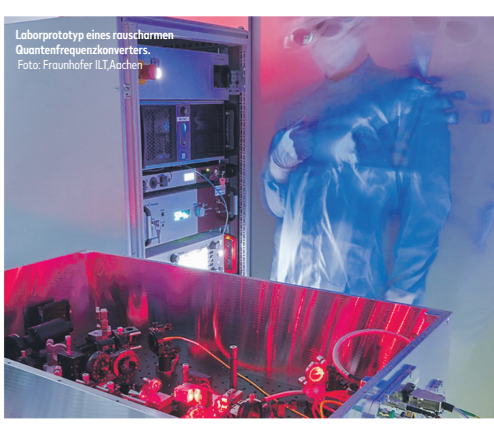
Laborprototyp eines rauscharmen Quantenfrequenzkonverters. Foto: Fraunhofer ILT Aachen
