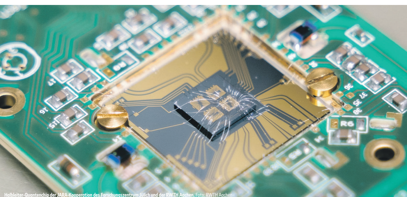
Halbleiter-Quantenchip der JARA-Kooperation des Forschungszentrum Jülich und der RWTH Aachen. Foto: RWTH Aachen
